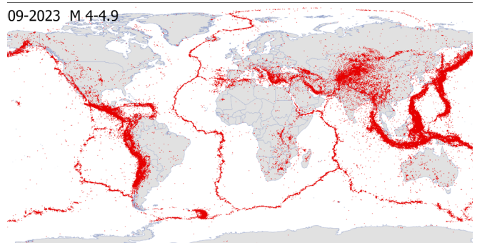
Terremotos M4,0-4,9 en el mundo durante 2009-2023
