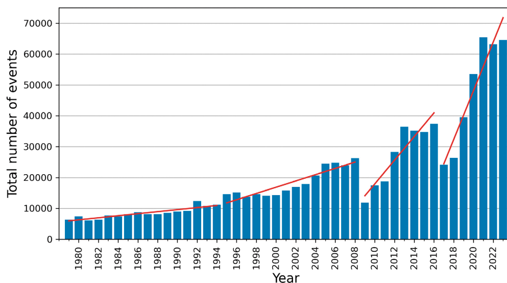
Terremotos M3-M9 en el mundo durante 1979-2023
