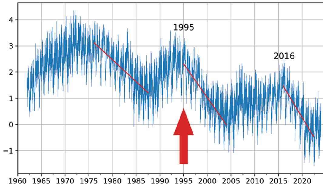
Desviación de la duración del día entre 1962 y 2023
