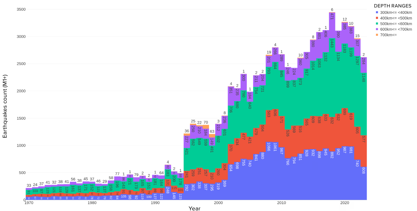
Terremotos de foco profundo M1+ en todo el mundo durante 1970-2023
