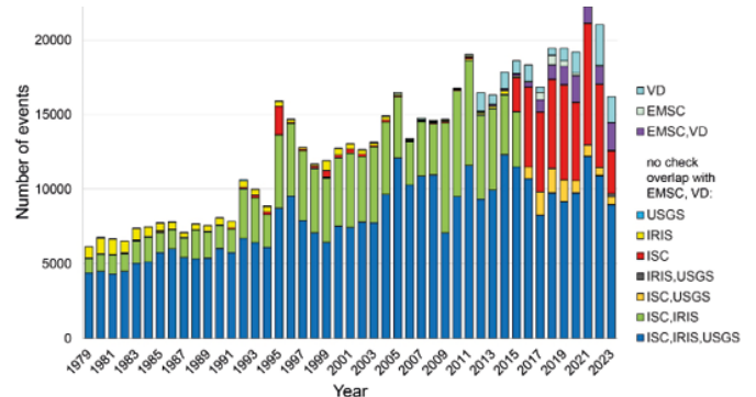
Número de eventos sísmicos únicos M4+ durante 1979-2023 notificados sólo por los servicios sismológicos indicados
